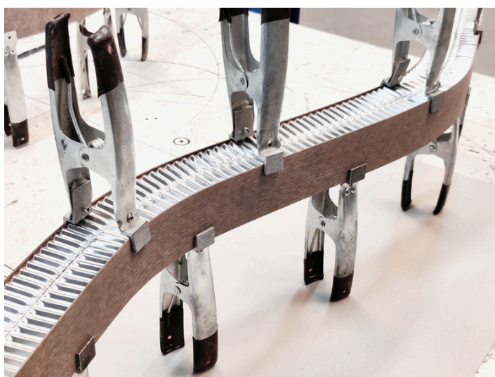
PreBeam® med laminat limet sammen
